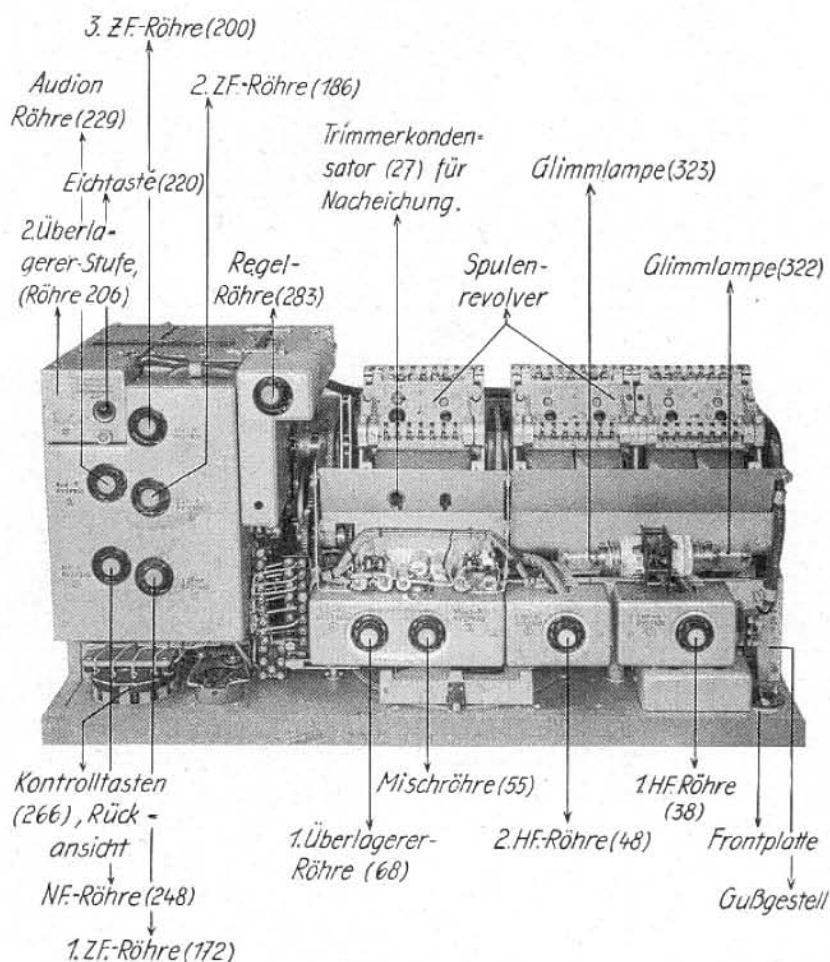
Abb. 2. Kurzwellen-Empfänger KwE a, ohne Kasten, Ansicht von oben
